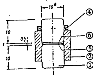
Εικόνα Ι3 Σύστημα κρούσης για ρευστά υλικά διαστάσεις σε μμ.
