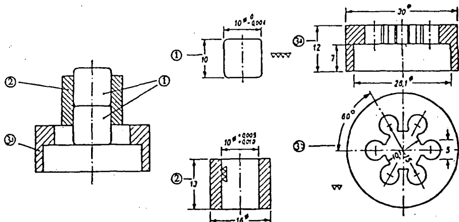
Εικόνα Ι2 Σύστημα κρούσης για κονιορτώδη ή ζυματώδη υλικά διαστάσεις σε μμ
