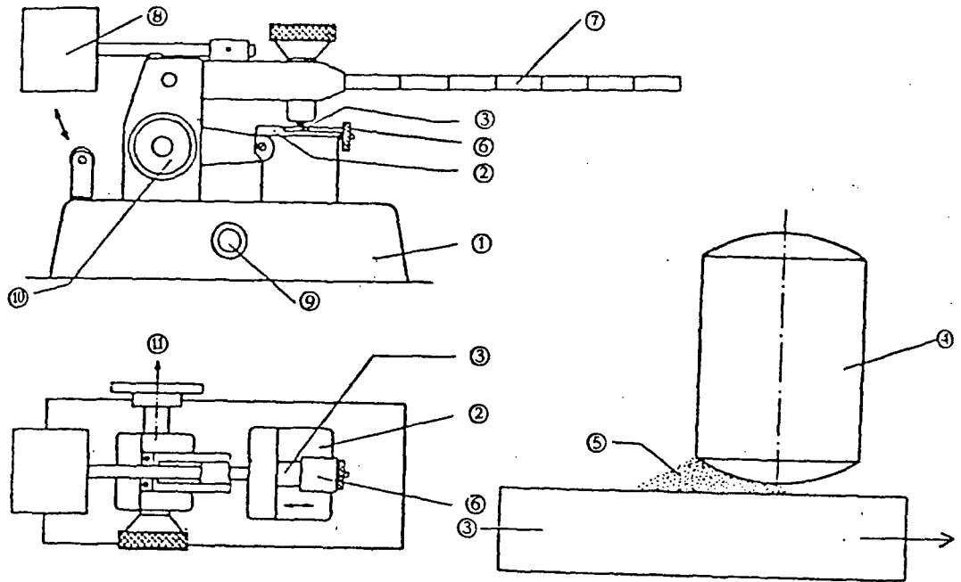
Εικόνα 14 Συσκευή τριβής
