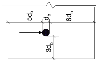
Σχ. Σ6.6: Ορισμός επικάλυψων βλήτρου
