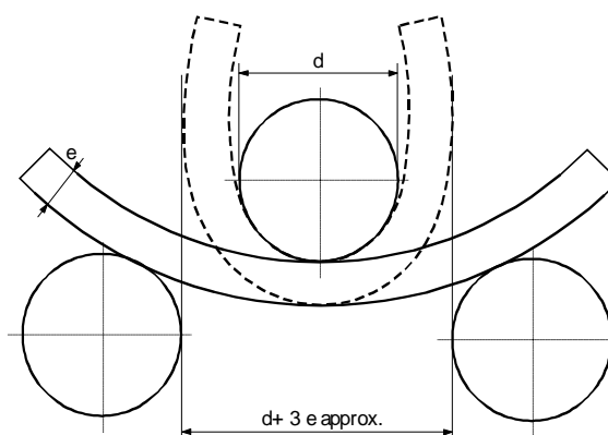
Διάγραμμα της δοκιμής κάμψης
