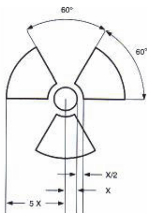
Βασικό σύμβολο τριφυλλίου με διαστάσεις βασισζόμενες σε έναν κεντρικό κύκλο ακτίνας X.
