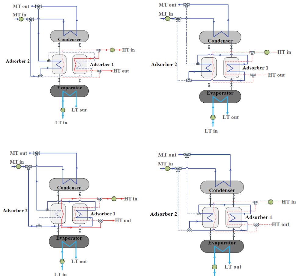
Σχήμα 27 Διαργασίες λειτουργίας ενός ψύκτη προσρόφησης
