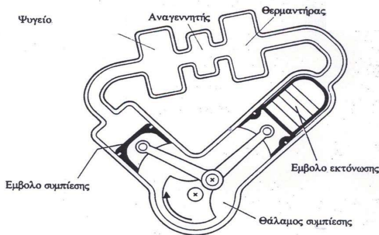
Σχήμα 18 Κινητήρας Stirling
