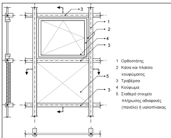
Σχήμα 4. Επιφάνειες τοιχοπετάσματος
