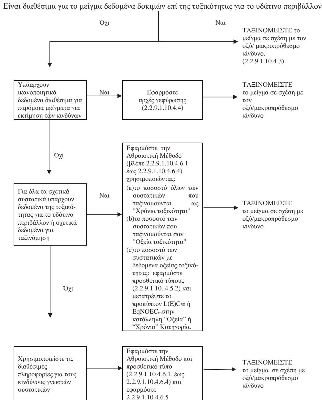
Σχήμα 2.2.9.1.10.4.2: Βαθμιδωτή προσέγγιση για ταξινόμηση μειγμάτων για οξείες και μακροπρόθεσμους υδάτινους περιβαλλοντικούς κινδύνους
