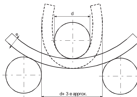
Σχήμα της δοκιμής σε κάμψη
